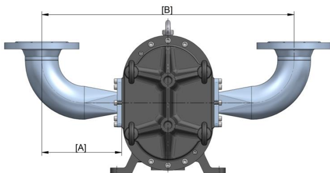
Bauform 2 | 90° Bogen oben in mm
