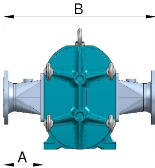
Bauform 1 Anschlussstutzen mit Anschlussflansch und O-Ring in mm / inches Design 1 Short, straight pipe connectors with connection flange and O-ring seal in mm / inches
