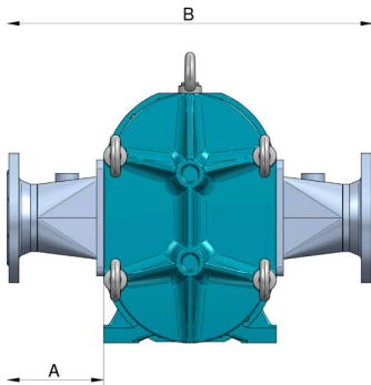
Bauform 1 Anschlussstutzen mit Anschlussflansch und O-Ring in mm / inches Design 1 Short, straight pipe connectors with connection flange and O-ring seal, in mm / inches
